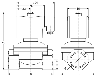
AR-2W21 32...50 мм
