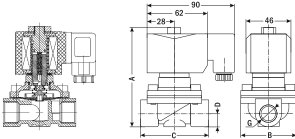
AR-2W21 12...25 мм
